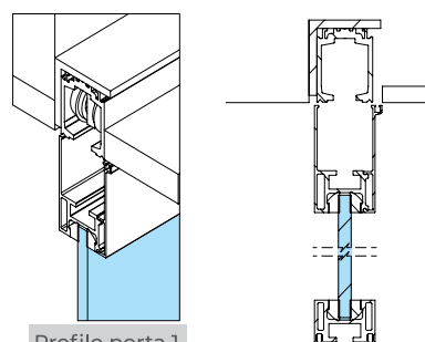
Profilo porta 1
