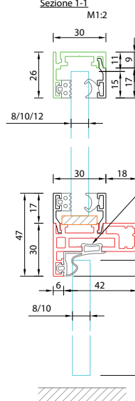
Section 1-1 Sezione 1-1
