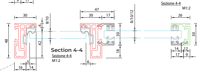
Section 4-4 Sezione 4-4
