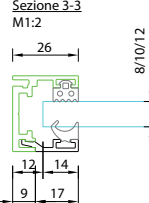
Section 3-3 Sezione 3-3
