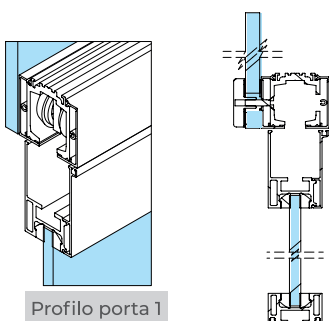
Profilo porta 1
