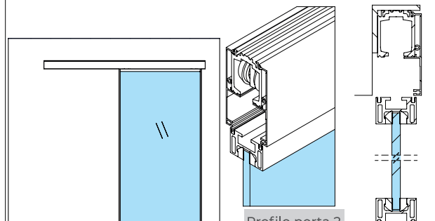
Profilo porta 2
