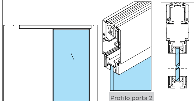
Profilo porta 2
