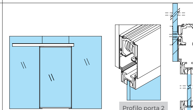
Profilo porta 2
