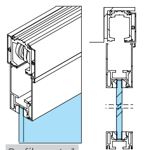
Profilo porta 1
